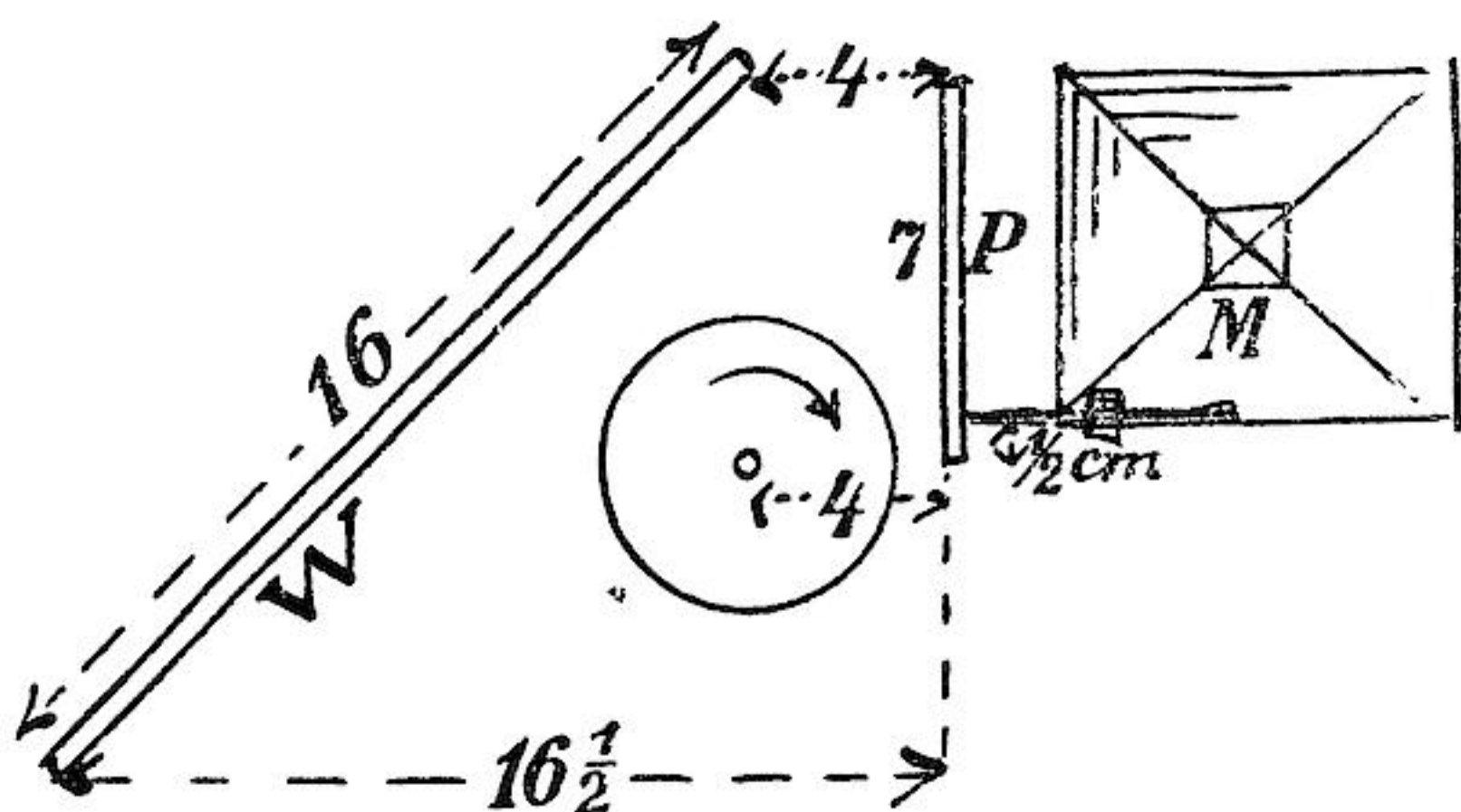
Fig. 27 a. Grundriß
